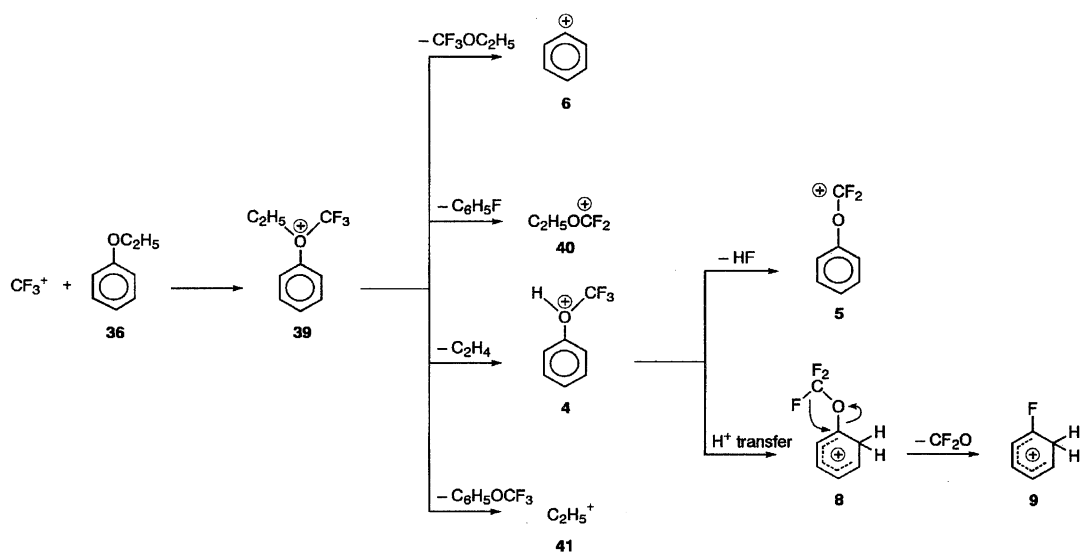
Scheme 14.
